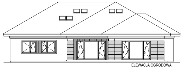
ELEWACJA OGRODOWA
