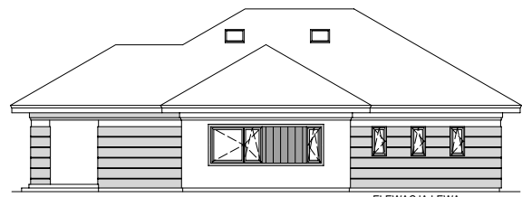
ELEWACJA LEWA
