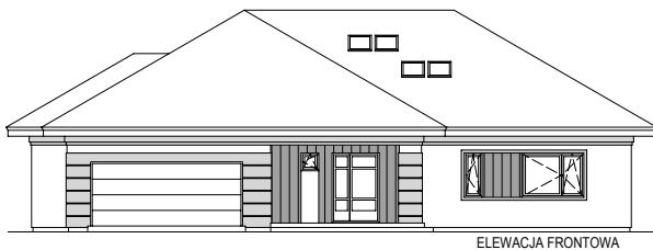
ELEWACJA FRONTOWA
